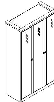
Шкаф 3-дверный распашной с зеркальными дверями МШг3-3/2 1312 x 590 x 2282
