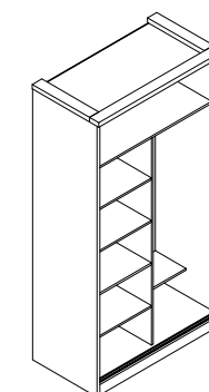
Внутреннее наполнение шкафов МШКг2-3.1/1 МШКг2-3.2/1
