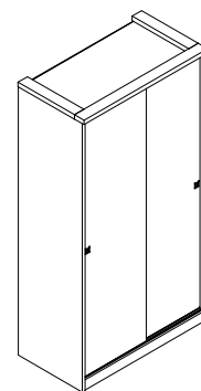
Шкаф-купе 2-дверный с глухими дверями МШКг2-3.1/2 1190 x 652 x 2282
