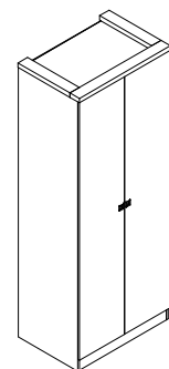
Шкаф 2-дверный распашной с глухими дверями МШг2-3/1 876 x 590 x 2282
