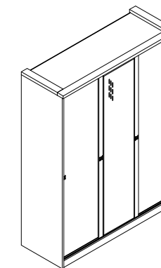
Шкаф-купе 3-дверный с 1 зеркальной дверью МШКг3-3.2/2 1726 x 652 x 2282
