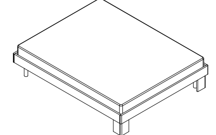
Кровать-тахта 2-спальная ТКПр-1600 1674 x 2070 x 362
