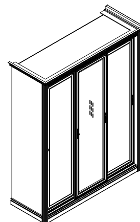
Шкаф-купе 3 дв. с 1 зеркальной дверью ТШКг3-3/2 1842 x 698 x 2307
