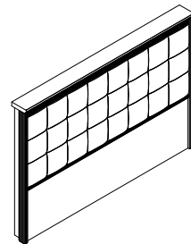
Панель стеновая на кровать с утолщением с мягкой вставкой ТПг-2/2 1782 x 160 x 1242
