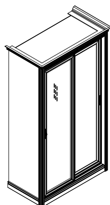
Шкаф-купе 2 дв. с 1 зеркальной дверью ТШКг2-3/2 1306 x 698 x 2307
